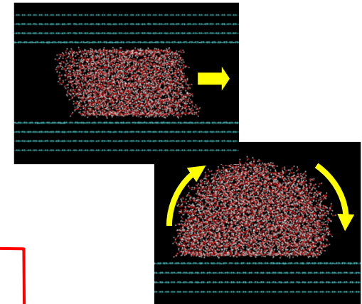
MPLナノ多孔体内の液滴輸送現象
