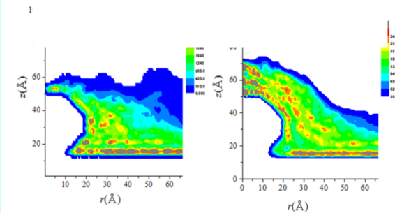
触媒層内のアイオノマーの酸素拡散現象
