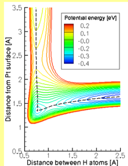
白金表面上での水素分子の解離吸着現象
