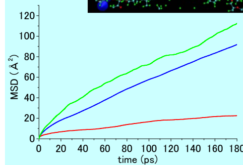
PEM内のプロトン輸送現象
