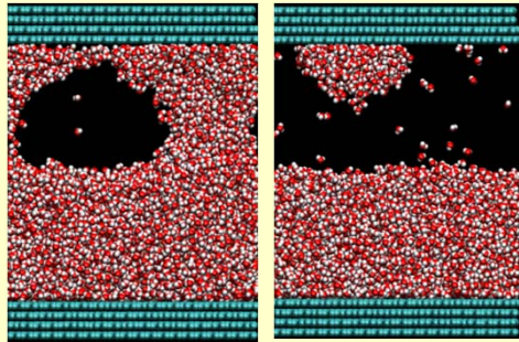
MPLナノ多孔体内の水分の蒸発・凝縮現象
