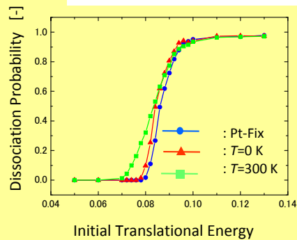
白金表面上での水素分子の解離吸着現象
